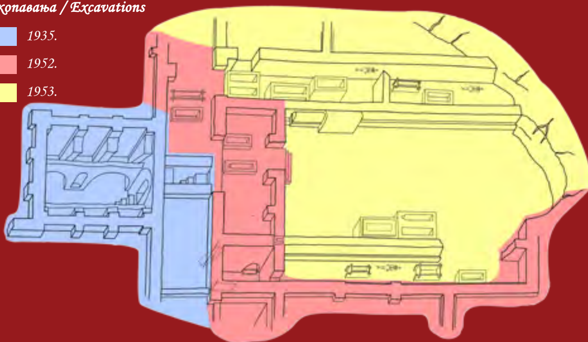
Сл. 10. Базилика са мучишницом, план (арх. В. Томашевић) Fig. 10. Basilica with martyrium, plan (arch. V. Tomasevic)
