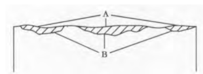
Локална корозија Local corrosion
